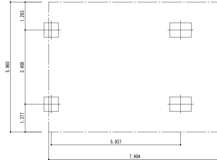
■ 基礎配置図
